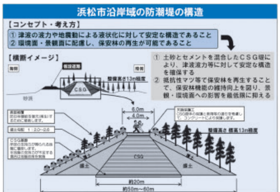
静岡モデルの「緑の堤防」の一つの施工事例
